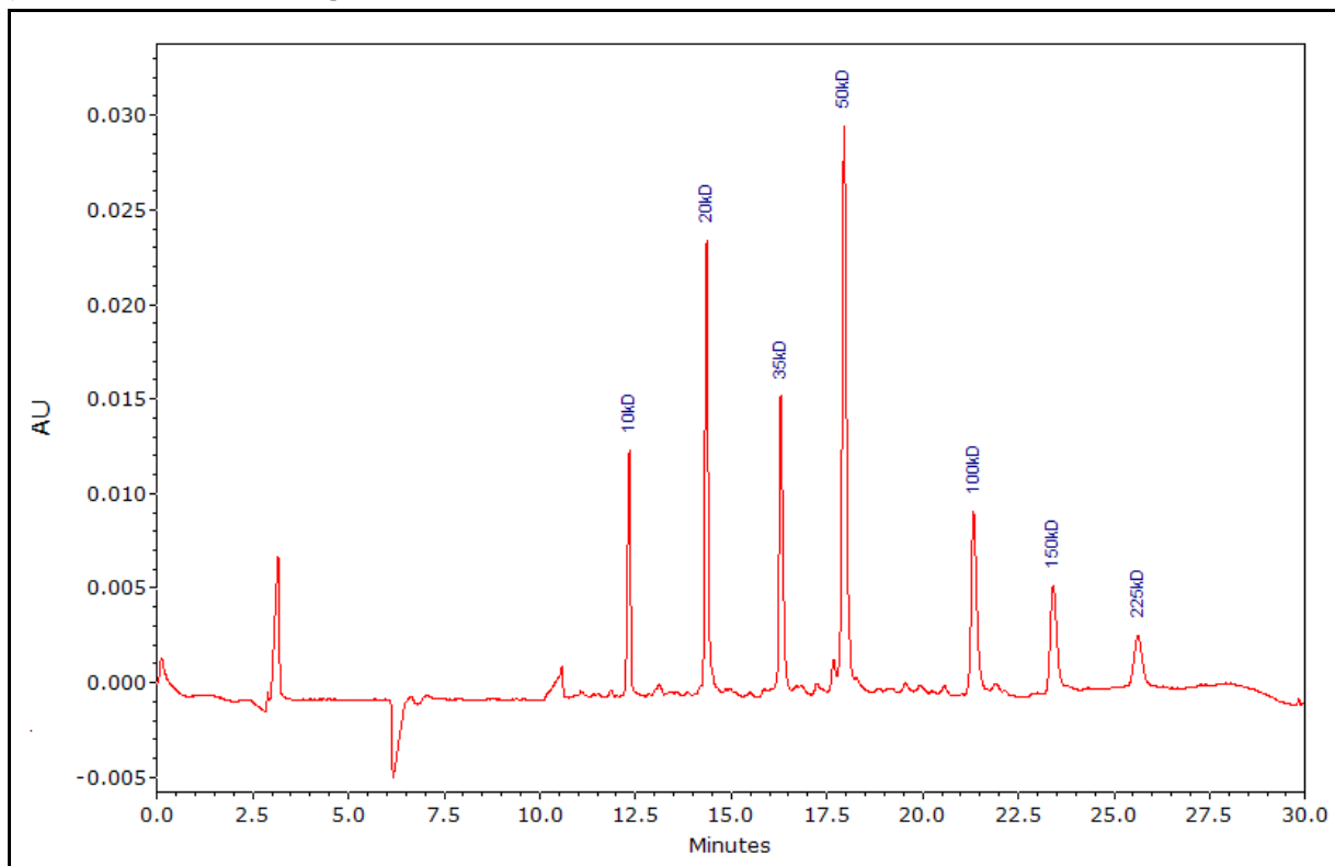
图 11 使用 SDS-MW Sample Buffer 的 SDS-MW Size Standard 分离
