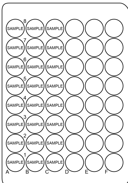
图 5 样品托盘布局
