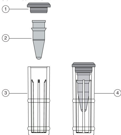
图 4 样品瓶安装
