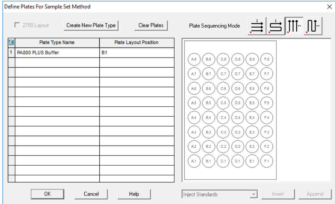
图 E.10 定义缓冲剂入口孔板之后
